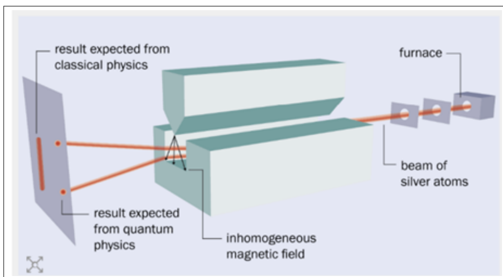
Figura 19: Rappresentazione schematica dell'esperimento di Stern-Gerlach
