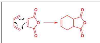
Figura 13: Esempio di reazione di Diels-Alder, notare il movimento a ruota degli elettroni
